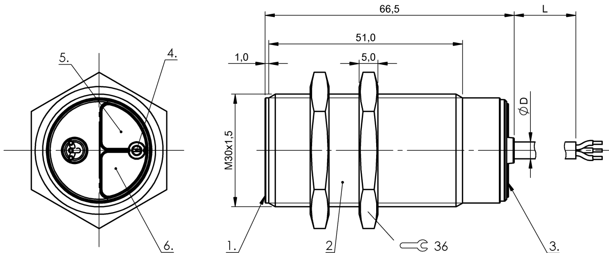
1) Face sensible 2) Boîtier 3) Couvreclre 4) Potentiomètre 5) LED de tension d'emploi 6) LED de visualisation d'état
