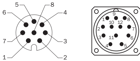
Vue du connecteur d'appareil M12/M23 sur le câble/boîtier
