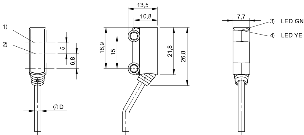
1) Axe optique récepteur 2) Axe optique émetteur 3) Tension d'emploi 4) Réception lumineuse
