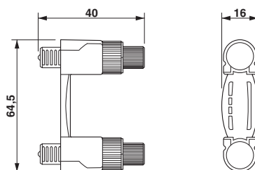
Dessin coté
