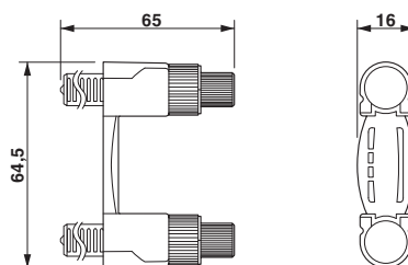
Dessin coté
