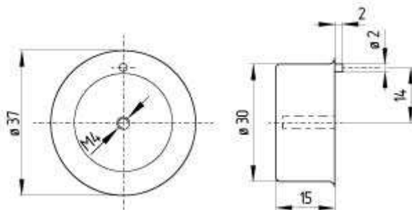
Plan d'encombrement (divers)
