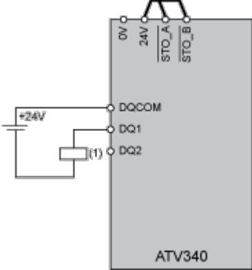
(1) Relais ou vanne
