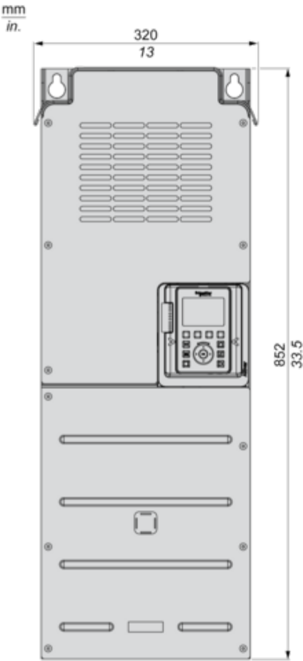
Variateurs sans capot supérieur IP21 Vues droite et avant
